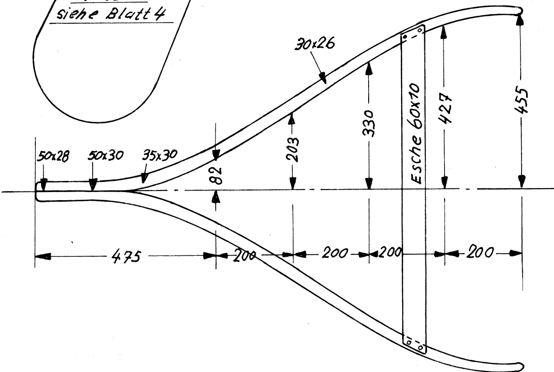
Gabelpinne 1:10 Material: Esche
